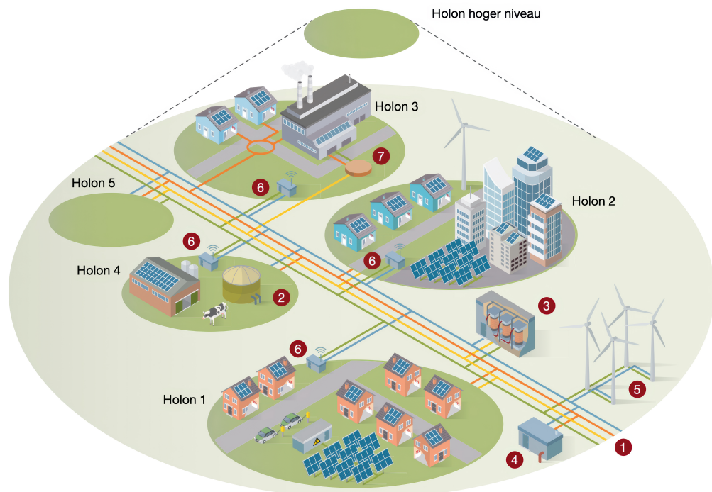
Figuur 19: Holarchische benadering van het energiesysteem.
