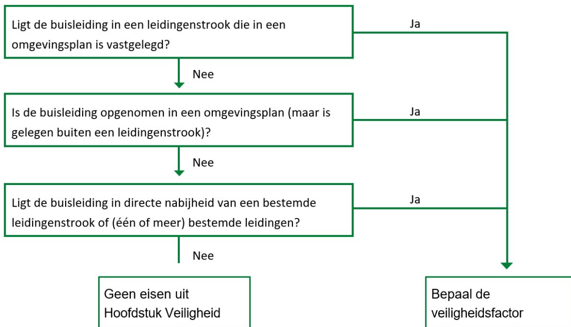
Figuur 3: Schema bepaling veiligheidsfactor
