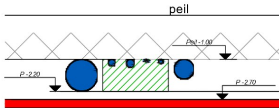
Figuur 2: beschikbare ruimte voor meerlaags leggen
