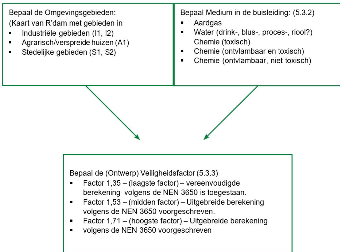
Figuur 4: Bepaling van de (Ontwerp) Veiligheidsfactor
