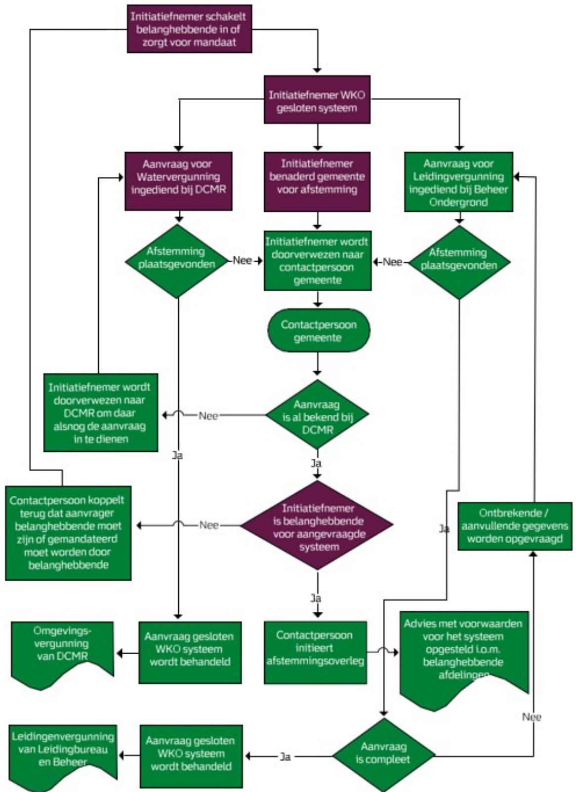
3.3.10 Proces open WKO systeem Paars = Exploitant Groen = LBBO/Provincie
