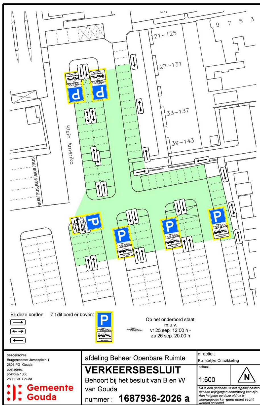
Situatietekening 1687936-2026 a
