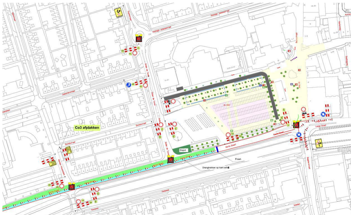
Situatieschets tijdelijke verkeersmaatregelen Urkerweg/Korte Dreef;
