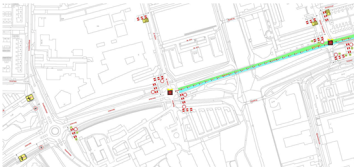
Situatieschets tijdelijke verkeersmaatregelen Urkerweg/Korte Dreef;
