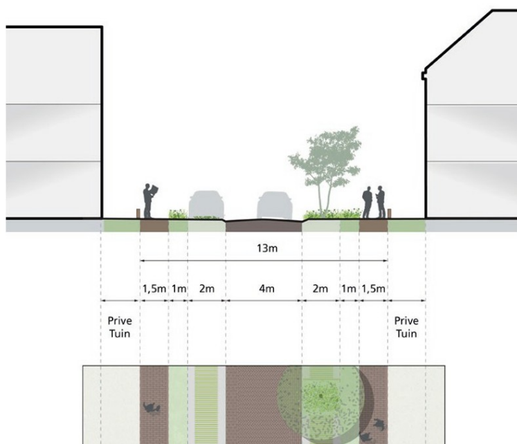
Afb. 155 - Profiel inrichting buurtontsluiting
