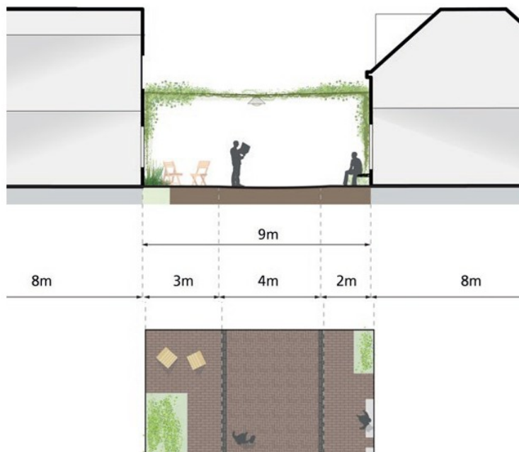
Afb. 1.56 - Profiel inrichting tussenstraten
