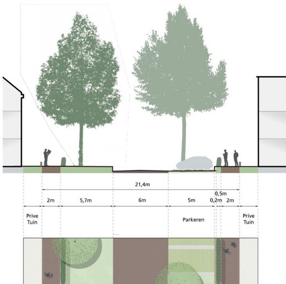
Afb.154 - Profiel inrichting hoofdontsluiting
