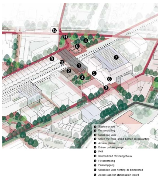
Figuur 47: principedetail stationsknoop
