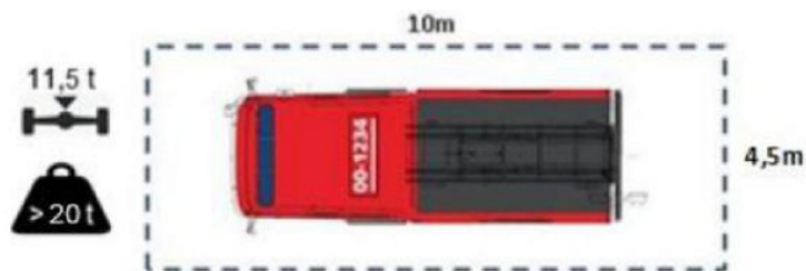
Figuur 7. Opstelplaats voor een tankautospuut
