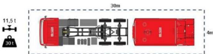
Figuur 9. Opstelplaats voor een grootwatertransportsysteem (haakarmchassis met dompelpompunit)
