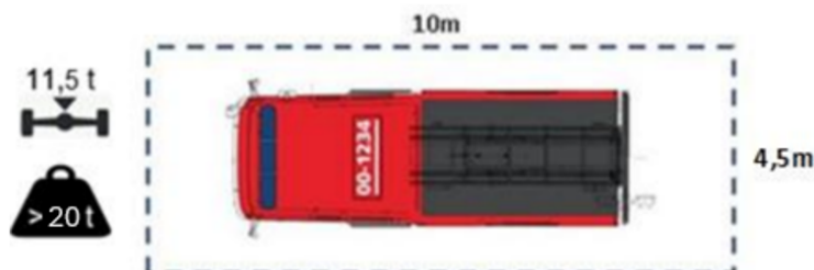
Figuur 7. Opstelplaats voor een tankautospuut
