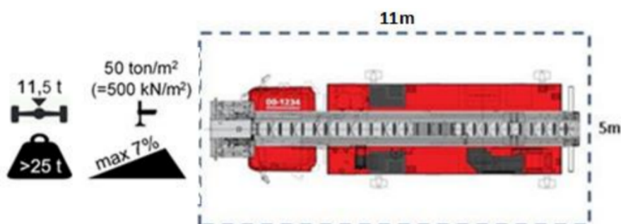
Figuur 8. Opstelplaats voor een redvoertuig
