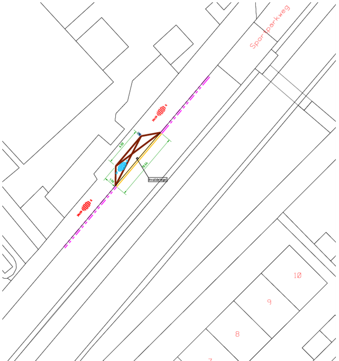
Afbeelding: aanlegtekening (schematisch) van de AGPP aan de Sportparkweg.
