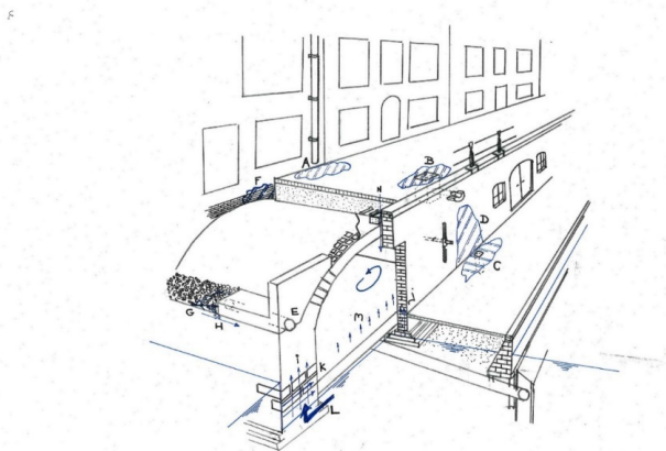
Figuur 6 - schets kelder met complexe vochtproblematiek; de bouwnaden (f) en (n) zijn de zwakste plekken
