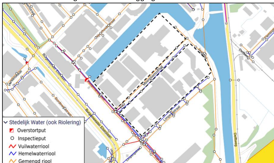
Figuur 38 Rioolstelsel in het plangebied
