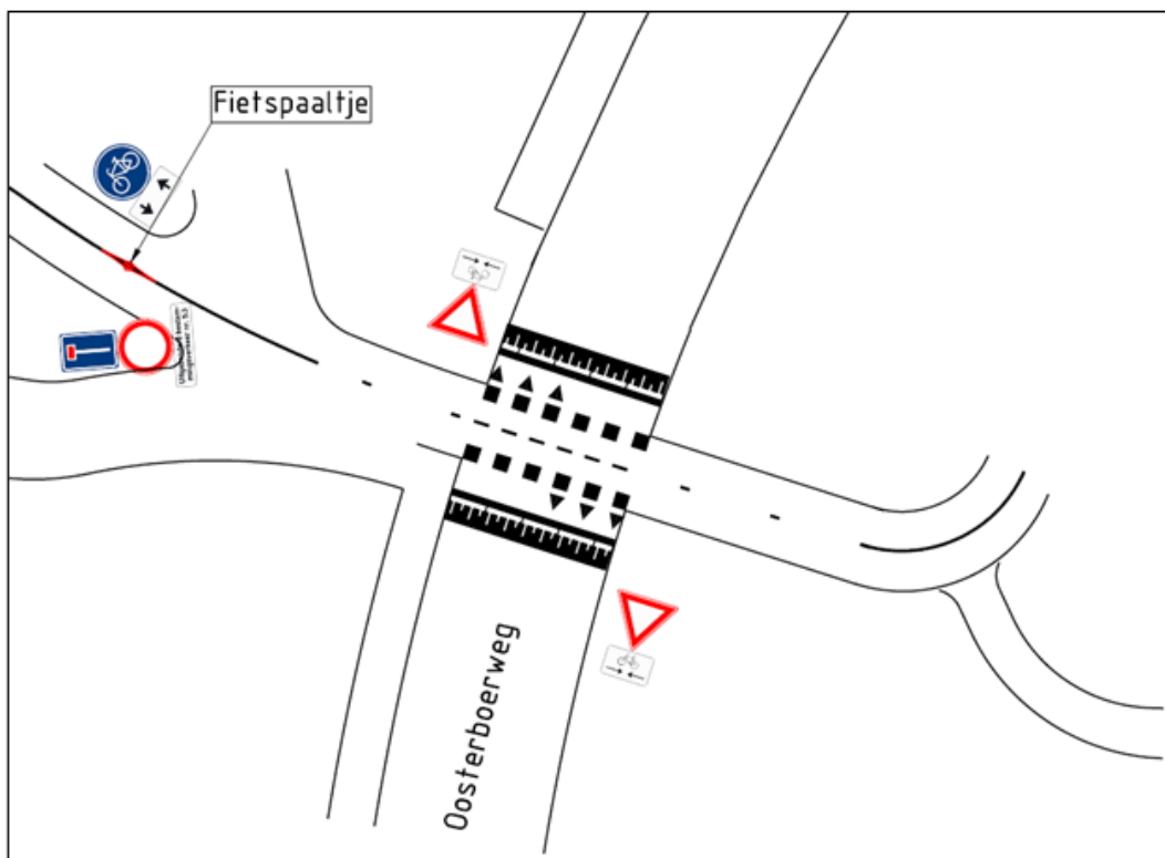
Situatietekening 2: Oostzijde, kruising Oosterboerweg
