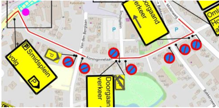
Situatieschets Koninginnelaan - Voorthuizen (Parkeerverbod)
