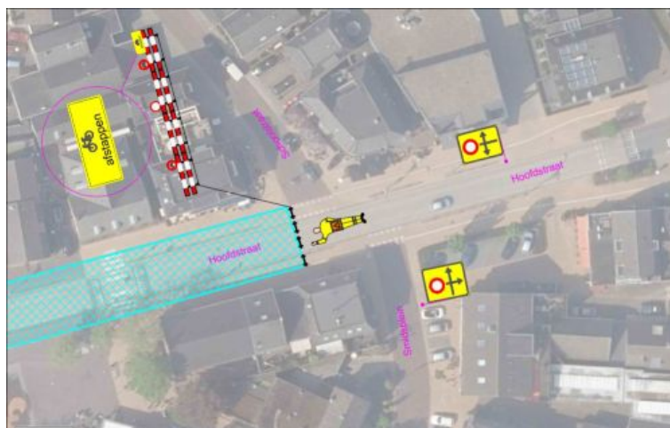
Situatieschets Hoofdstraat/Schoolstraat - Voorthuizen (inrijverbod)
