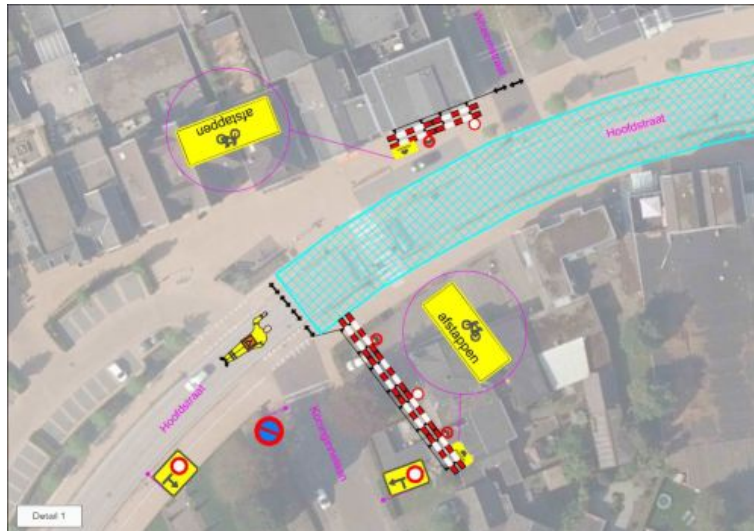
Situatieschets Hoofdstraat/Koninginnelaan - Voorthuizen (inrijverbod)
