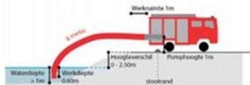
Figuur 4.14: Opstelplaats voor bluswater-winning van open water
