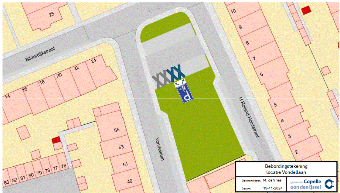
Bebordingstekening Vondellaan ter hoogte van huisnummer 55
