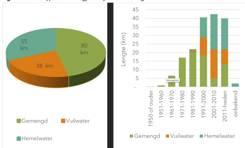
Figuur 3. Stelseltypen en aanlegjaar vrijverval riolering
