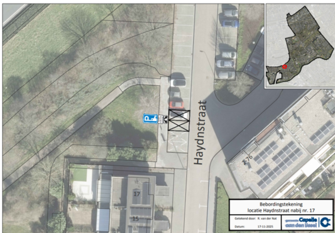
Bebordingstekening locatie Haydnstraat nabij nummer 17
