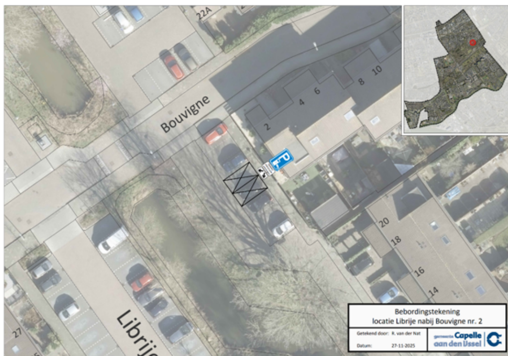
Bebordingstekening locatie Librije nabij Bouvigne nummer 2
