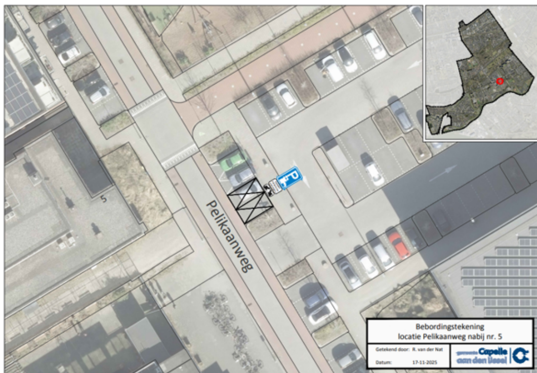
Bebordingstekening locatie Pelikaanweg nabij nummer 5
