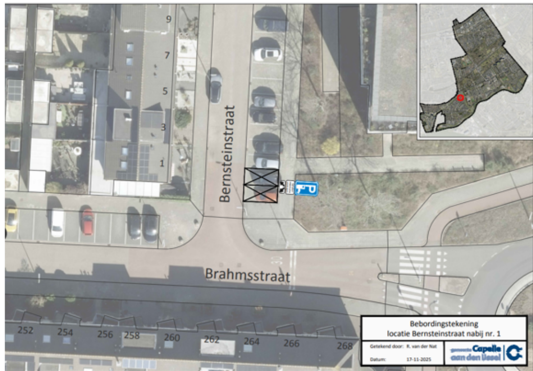
Bebordingstekening locatie Bernsteinstraat nabij nummer 1
