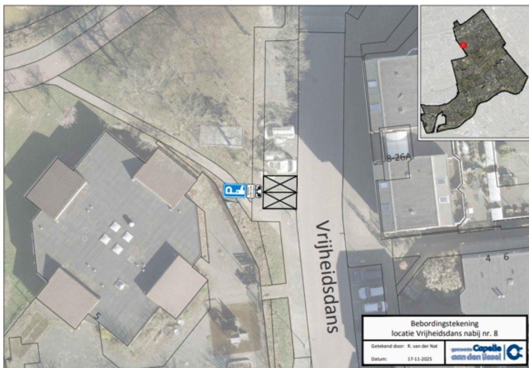
Bebordingstekening locatie Vrijheidsdans nabij nummer 8
