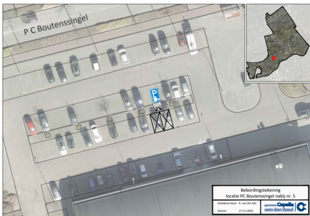
Bebordingstekening locatie PC Boutenssingel nabij nummer 5
