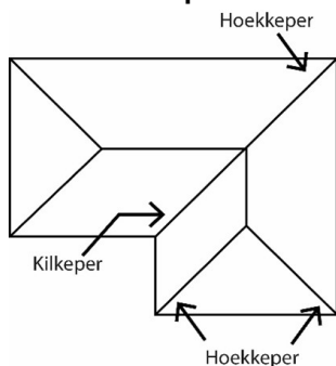
Afbeelding 2: hoek- en kilkeper
