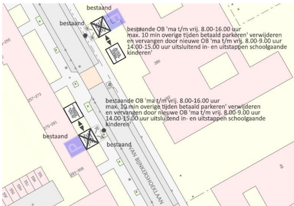
Uitsnede uit bebordingsplan
