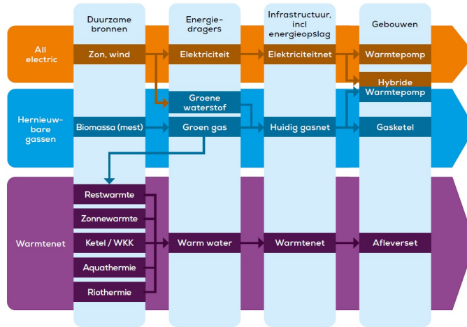
Warmtealternatieven stromenschema
