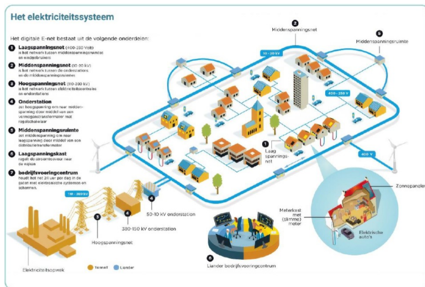
Figuur 1: visuele weergave van het elektriciteitssysteem.
