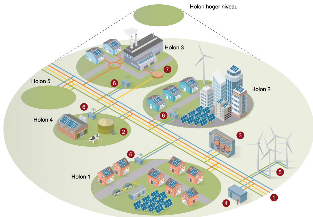
Figuur 20: Holarchische benadering van het energiesysteem.
