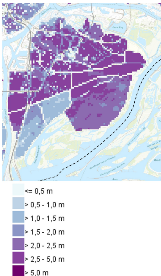
Figuur 22 - Overstromingsbeeld primaire kering
