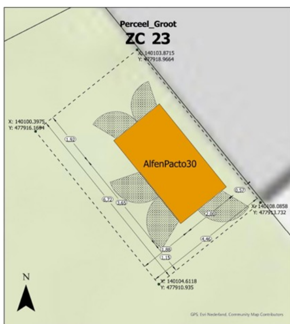
Situatie schaal: 1:50
