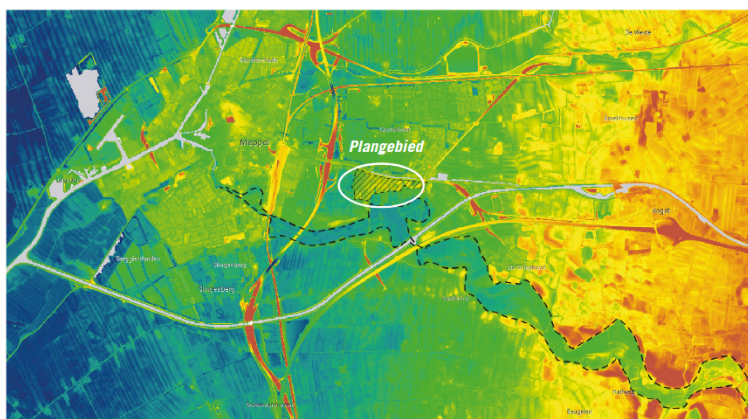
Hoogteverloop Meppel oost. Rood is hoog, blauw is laag. Het Reestdal is goed zichtbaar.
