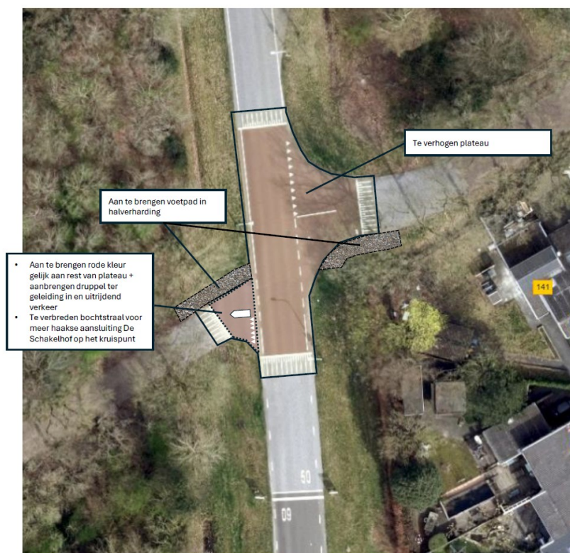
Bijlage 4 – Schematisch overzicht infrastructurele maatregelen
