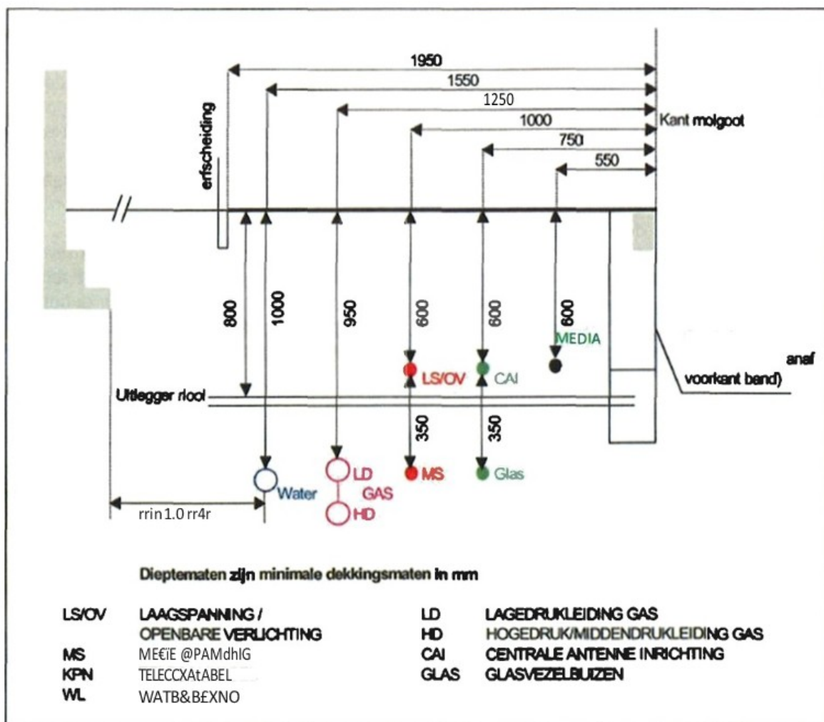
Figuur 1: standaard dwarsprofiel
