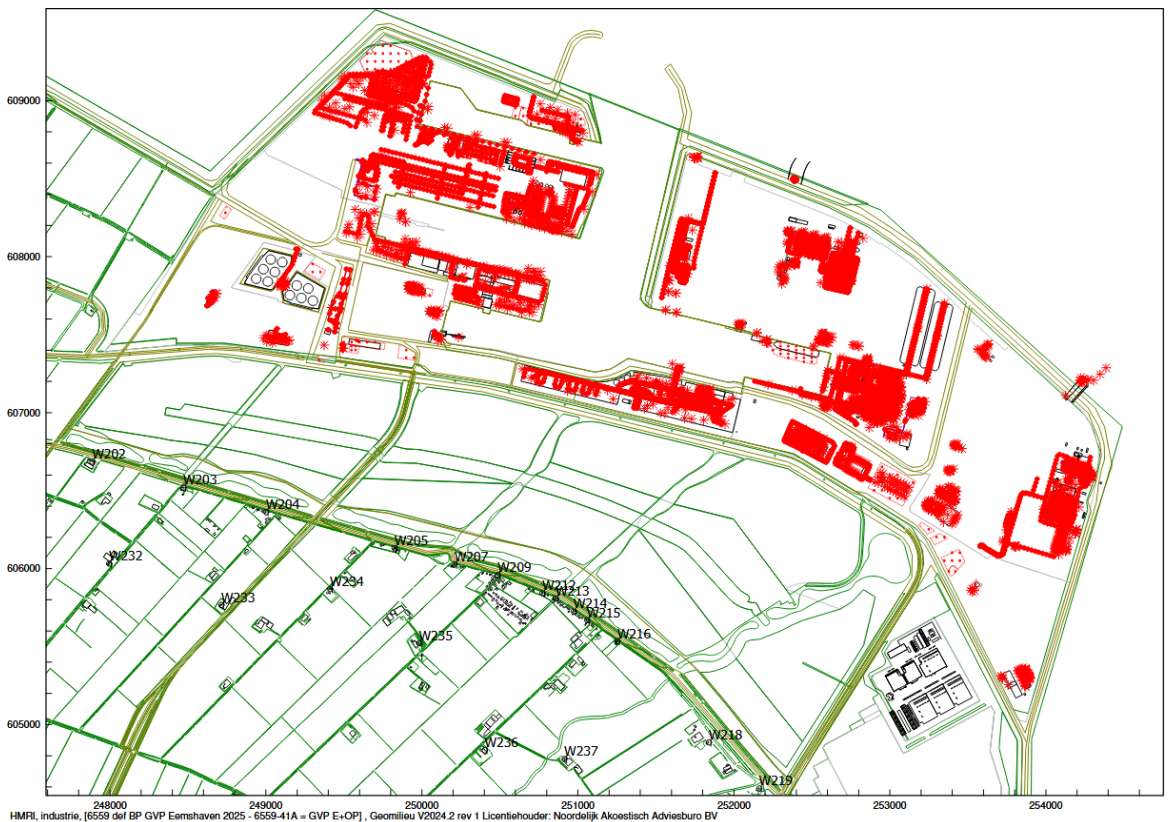
Detail geluidverdeelmodel: Eemshaven vergunde bronnen
