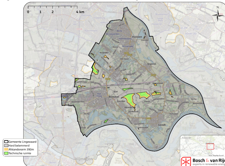
Figuur 3 Ruimte voor windturbines met tiphoogte 195 meter
