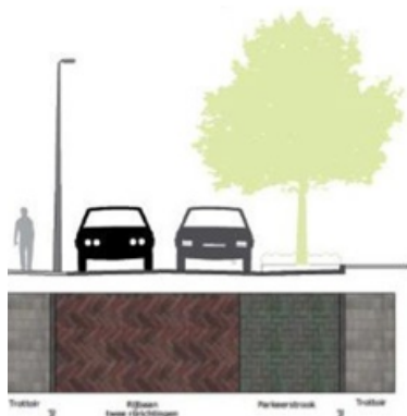
Woonstraat Standaard wegprofiel (conform lior)
