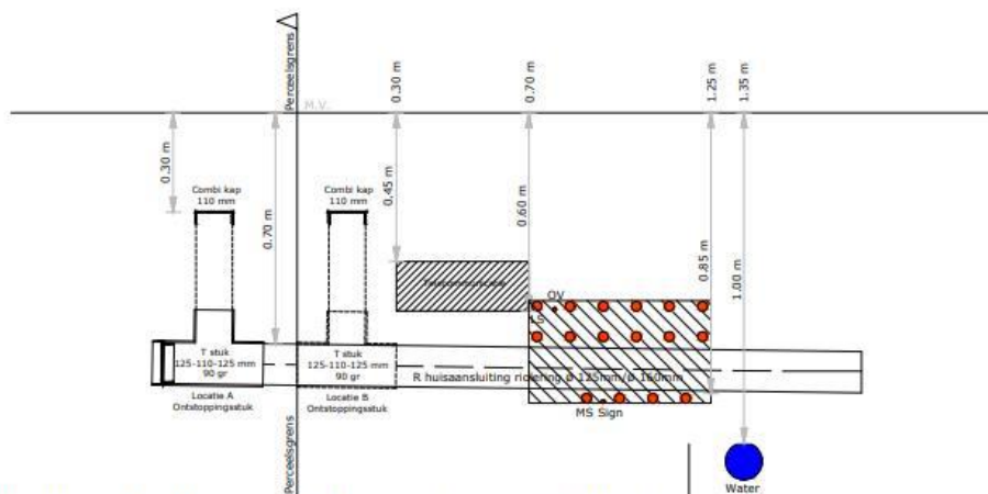
Kabel en leiding profiel zonder gasleiding
