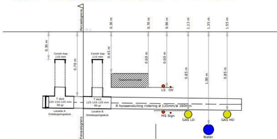
Kabel en leiding profiel standaard
