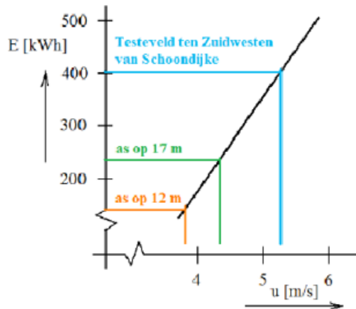
Figuur 7.2: Jaarlijkse energieopbrengst E [kWh] per vierkante meter rotoroppervlak op 12 [m], op 17 [m] ashoogte bij de verwachte windsnelheid. Bron: Ingrenious 2012, Resultaten testveld kleine windturbines Schoondijke
