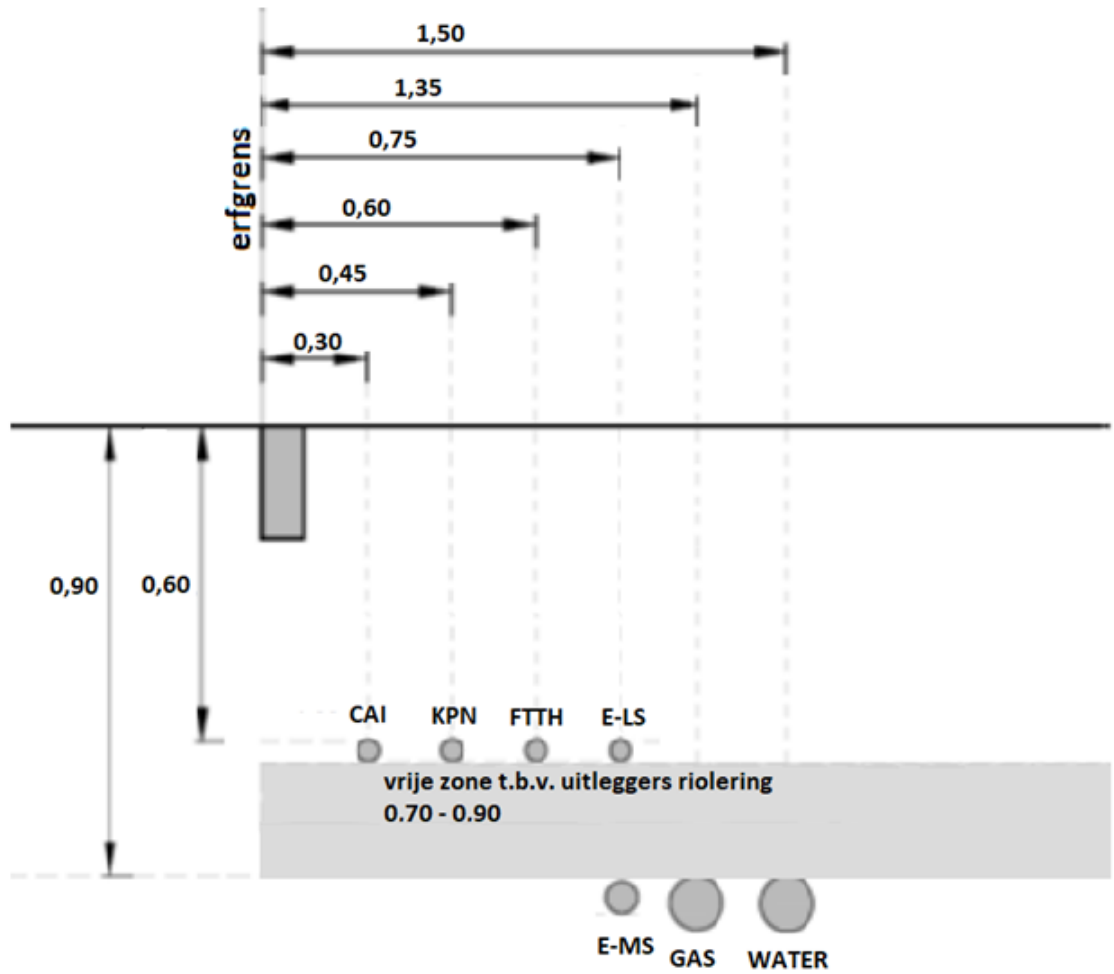
Figuur 1 - Standaard dwarsprofiel 01 (FTTH en telecom)
