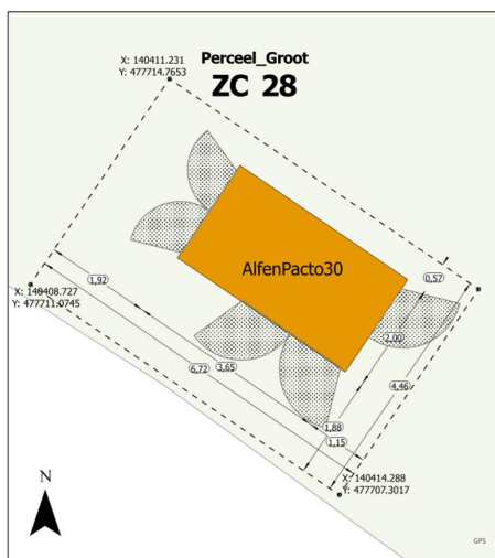
Situatie schaal: 1:45
