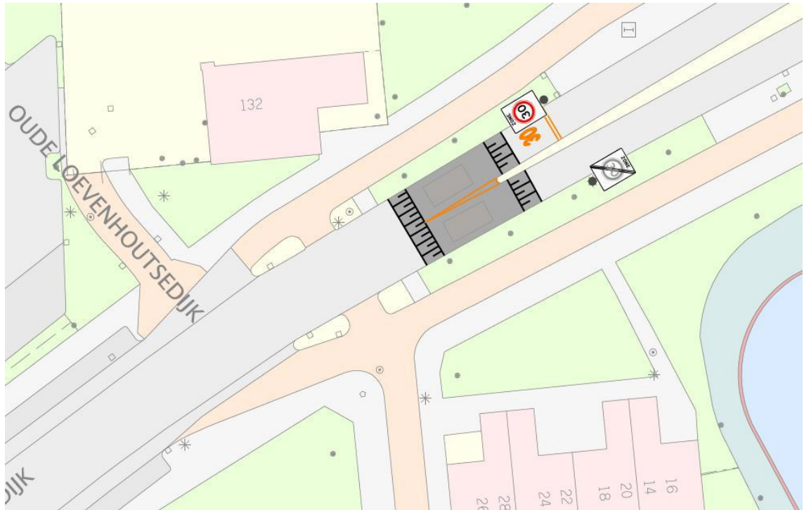
Uitsnede bebordingsplan
