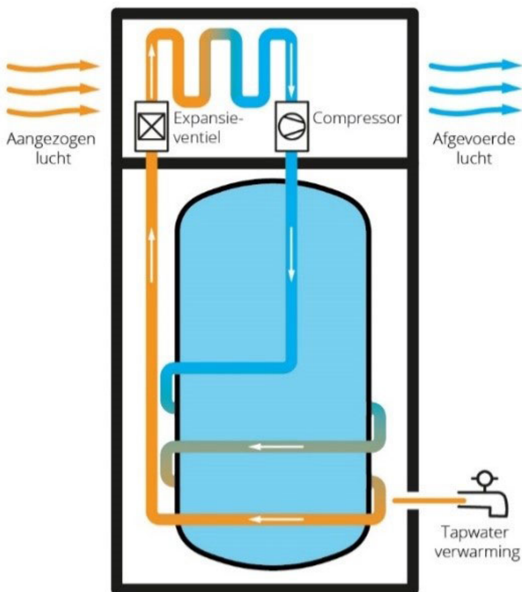
Figuur 8: Warmtepompboiler
