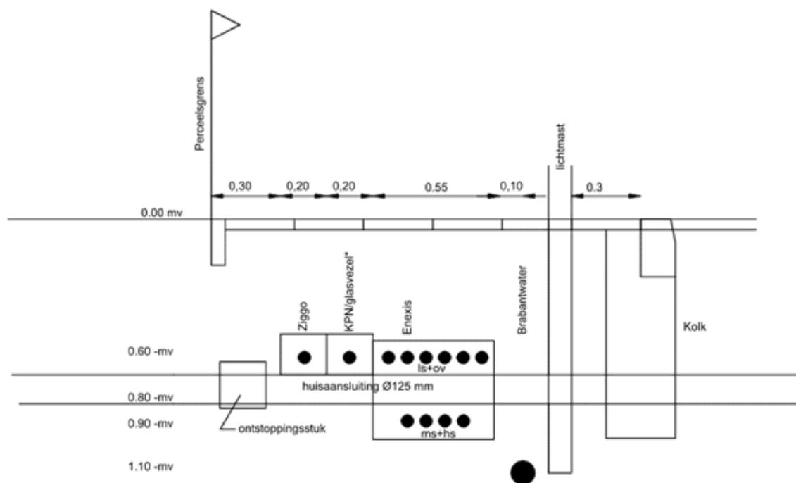
Principe dwarsprofiel
