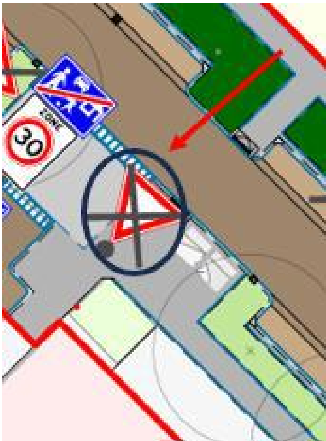
Uitsnede bordenplan
