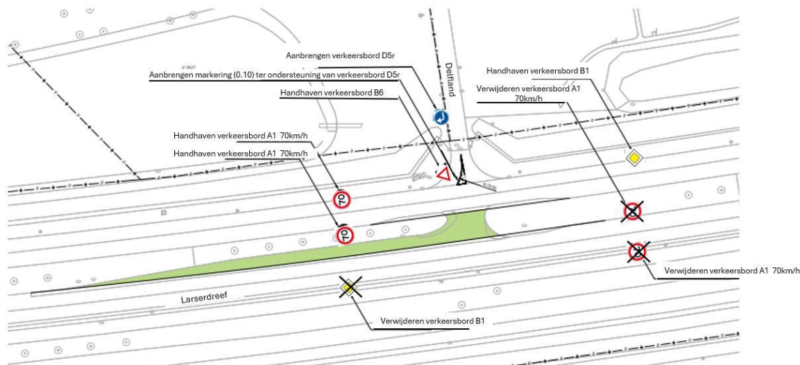
Tekening bij verkeersbesluit (registratienummer: 250005830) aanpassing kruispunt Larserdreef-Delfland; afsluiten middenberm Larserdreef
