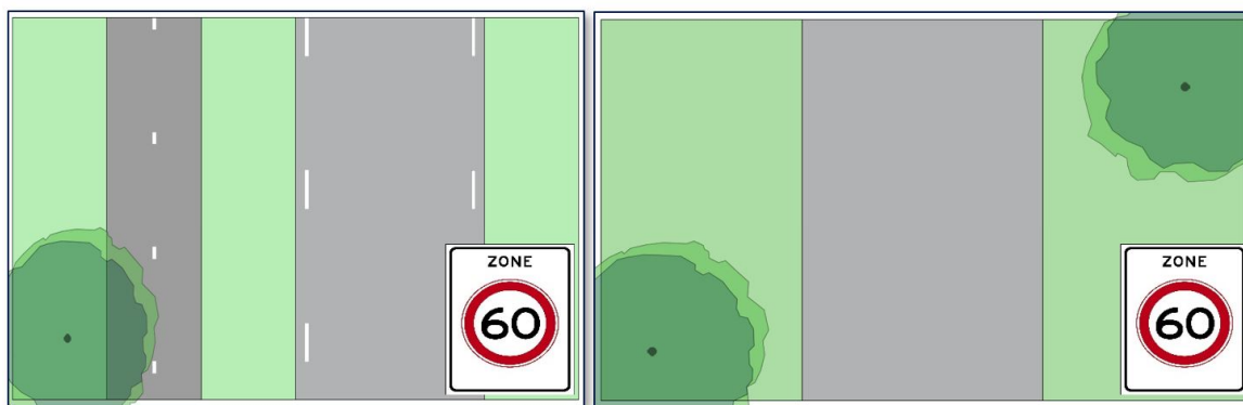
Figuur 9: Ideale inrichting erftoegangsweg buiten de bebouwde kom
