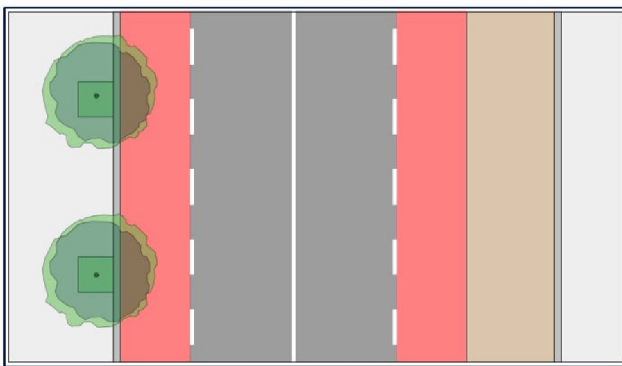
Figuur 7: Inrichting gebiedsontsluitingsweg 30
