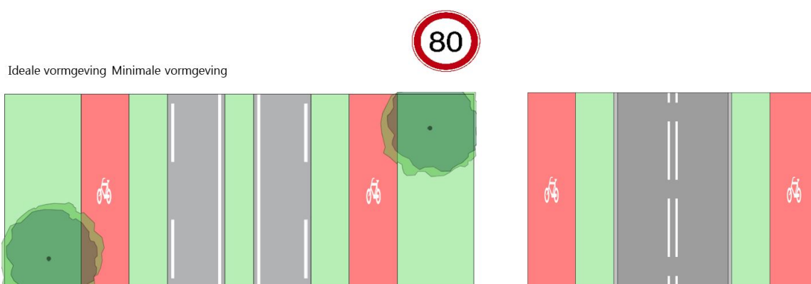
Figuur 4: Ideale/ minimale inrichting gebiedsontsluitingsweg buiten de bebouwde kom
