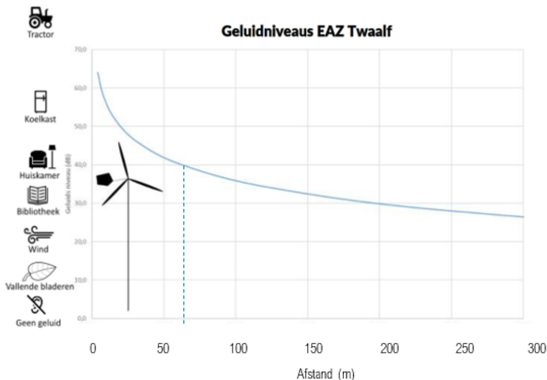
Figuur 6.2 Verhouding geluidsniveau kleine windturbine EAZ Twaalf met alledaagse geluidsbronnen t.o.v. afstand in meter. Op een afstand van 60 meter bedraagt het geluidsniveau van de EAZ Twaalf rond 40dB. Bron: EAZ twaalf informatieblad
