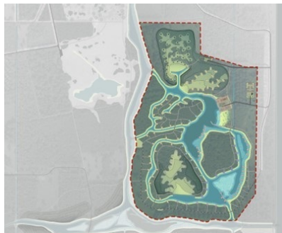
Figuur 2.3 Situatietekening van de voorgenomen situatie
