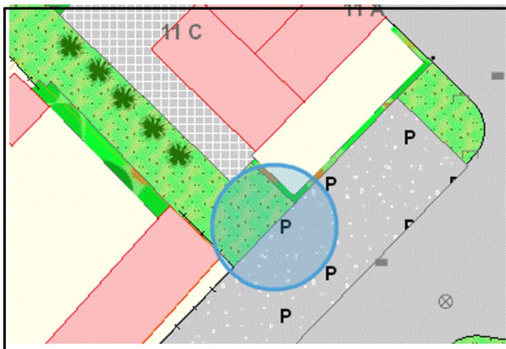
Bovenaanzicht
