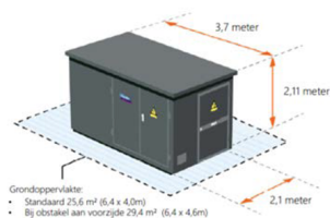
Afmetingen trafo
