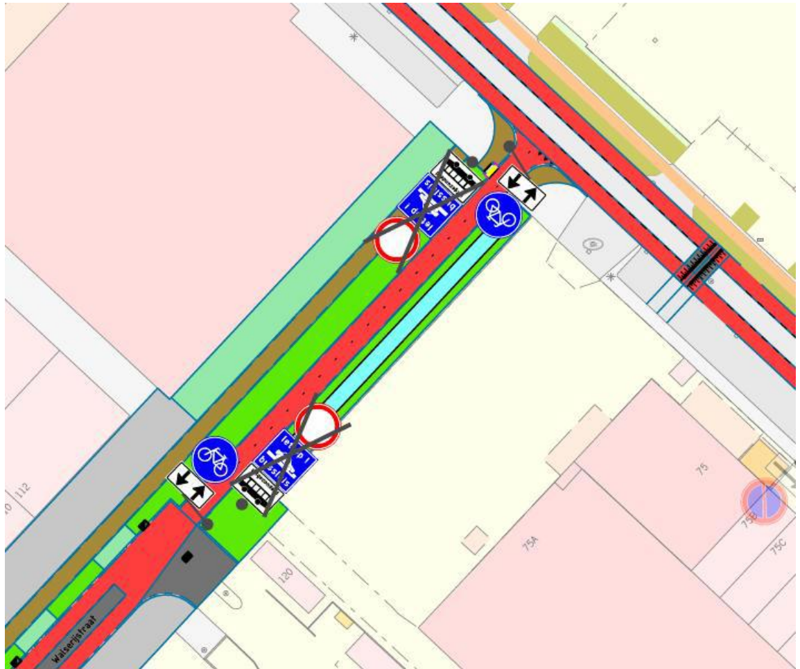
Uitsnede bordenplan
