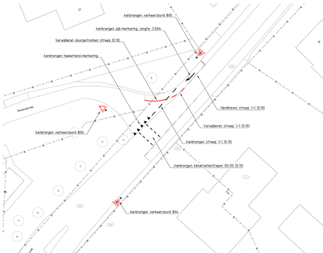
Kruispunt Boxbergerweg – Bevrijdingsweg
