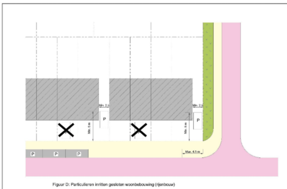
Figuur D Particuliere inritten gesloten woonbebouwing (rijenbouw)
