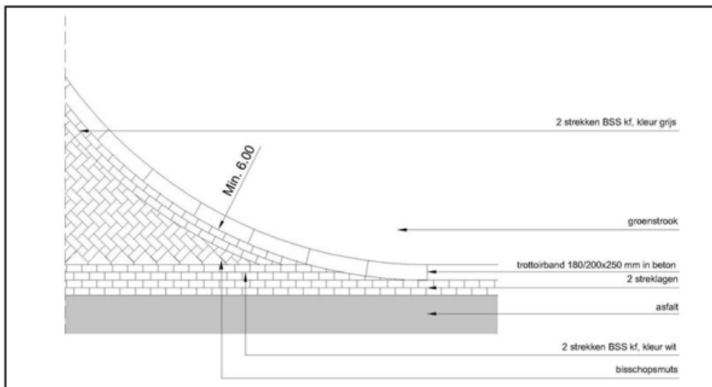
Standaard inritconstructie t.b.v. bedrijfsmatig gebruik type 2
