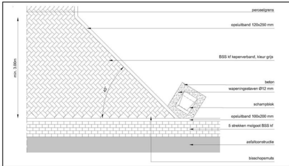
Standaard inritconstructie t.b.v. bedrijfsmatig gebruik type 1
