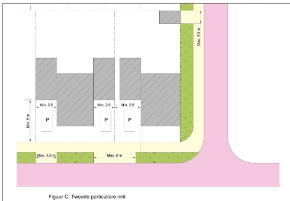
Figuur C Tweede particuliere inrit
