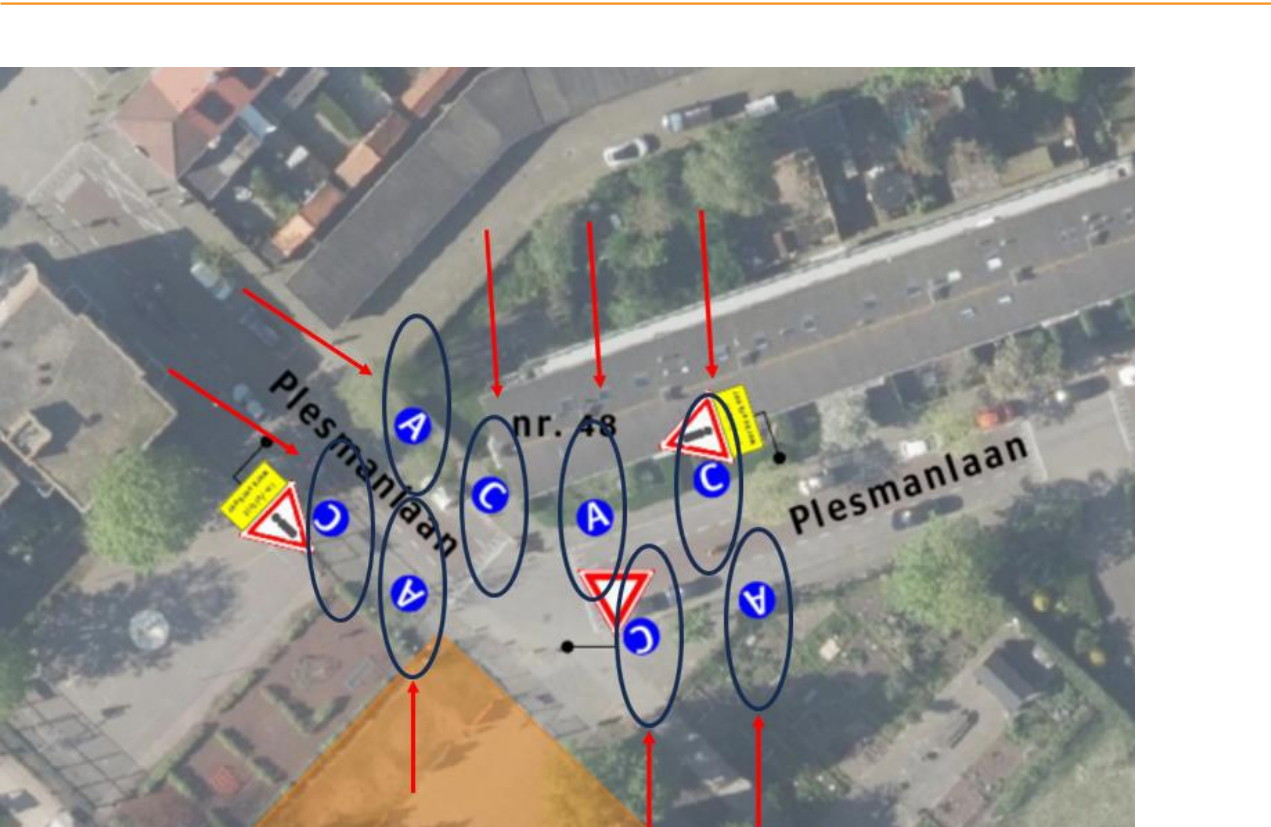
Uitsnede bordenplan
