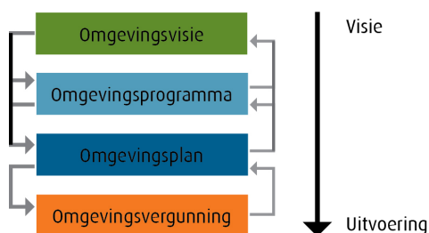
Figuur 47 Instrumenten omgevingswet
