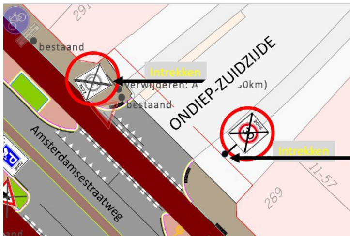
Uitsnede bebordingsplan
